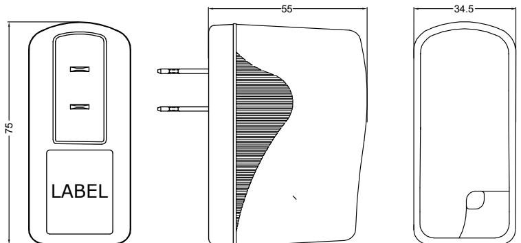
UNIVERSAL INPUT
